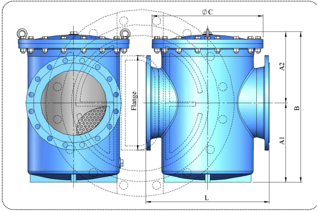
DIMENSIONS
